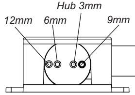
Wahl des Hubs mittels der Position des Bolzens
